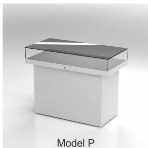
Model P Ganzglas-Tischvitrine mit zurückspringendem Sockelunterbau Table Case with retracted base plinth
